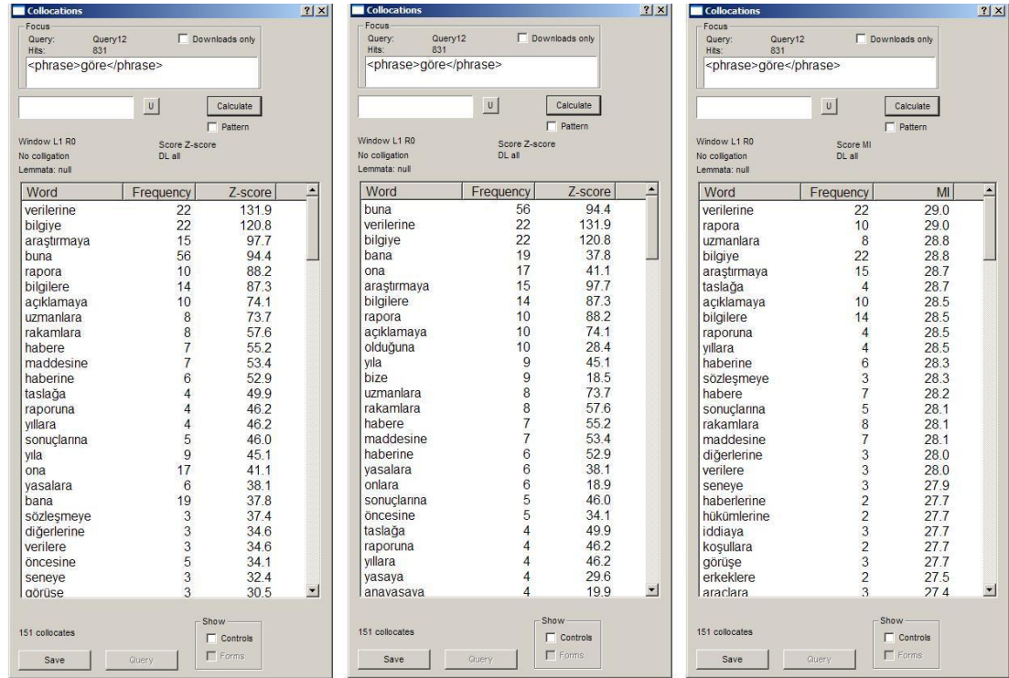
Şekil (2) Xaira ile eşdizim çözümlemesi. Sırasıyla Z-puanı, eşdizim sıklığı ve MI puanına göre sıralama
