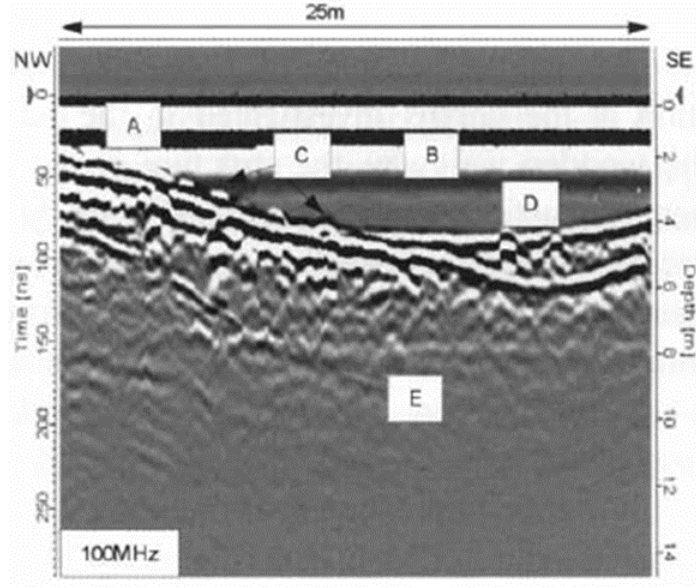
Şekil 3.14 A: Köprüden kaynaklı herhangi bir gürültü bulunmamaktadır, B: Ringing ya da tekrarlı yansıma, C: Jet ski koltuğu ve benzin kutusu, D: Göl tortusunda kısmen batmış belirtiler, E: Sediman ve anakaya sınırı (Ruffell 2006)
