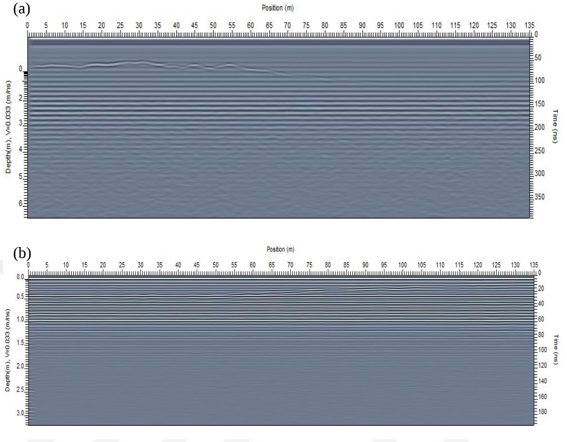
Şekil 4.7 100 MHz (a) ve 500 MHz (b) önceki veri işlem adımına ek medyan filtre uygulanmış WPR kesitleri
