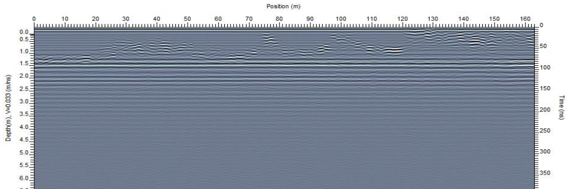
Şekil 3.24 Bant geçişli süzgeç uygulanmış WPR kesiti
