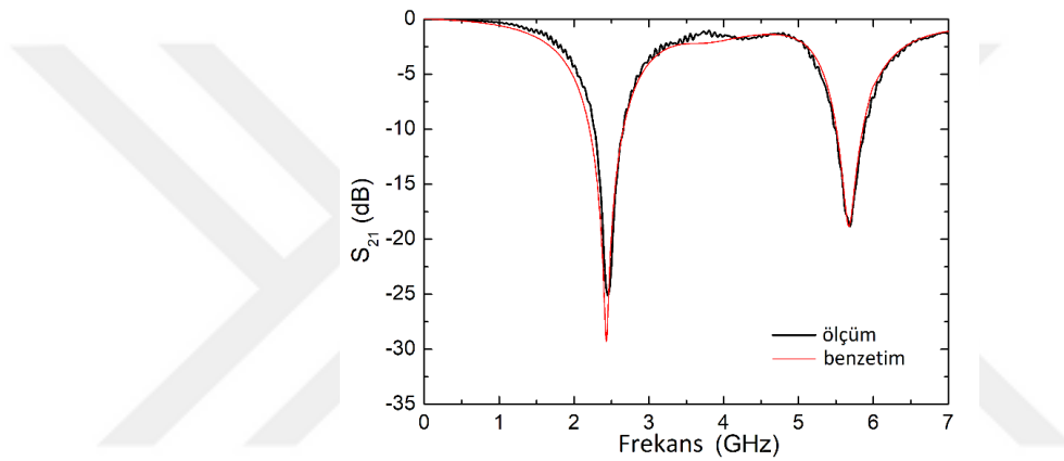
Şekil 4.25 Üretilen boş sensörün ölçülen iletim spektrumu ve benzetim sonuçlarıyla karşılaştırılması
