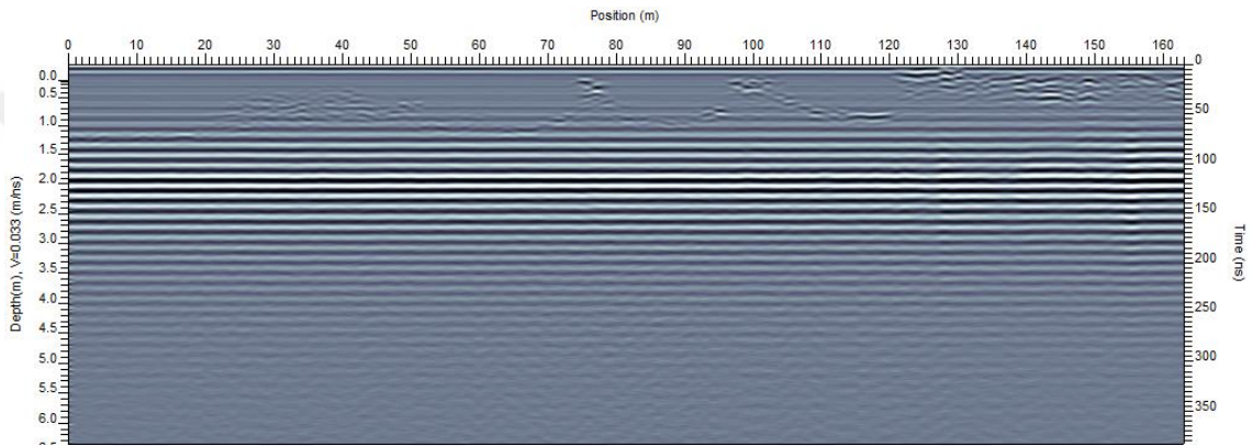
Şekil 3.20 Başlangıç zamanı düzeltmesi uygulanmış WPR kesiti
