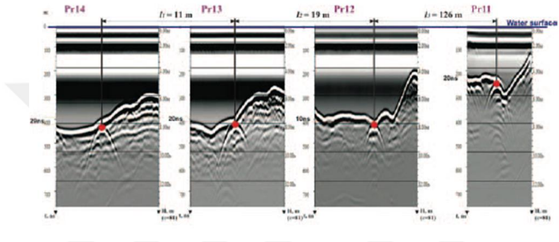
řekil 3.10 14, 13, 12 ve 11. Profillere ait iřlenmiř radargramlarda boru anomalisinin grntlenmesi (Khristoforov vd. 2016)
