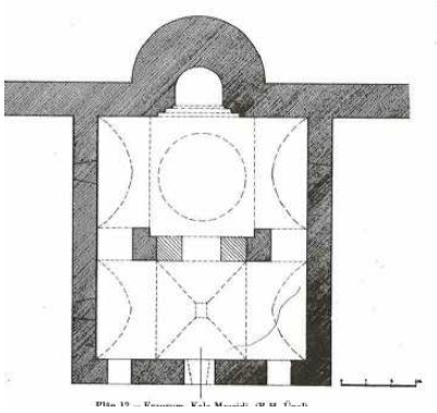
Çizim.1: Kale Mescidi Planı
